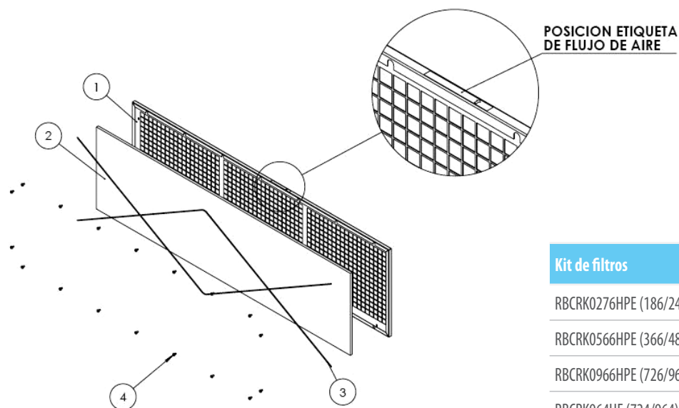
DETALLE B ESCALA 1 : 3
