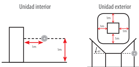
Medición presión sonora - Standard JIS B8616-2006
