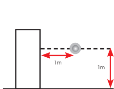
Medición presión sonora - Standard JIS B8616-2006
