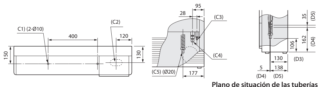
Plano de situación de las tuberías
