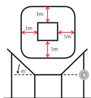
Medición presión sonora - Standard JIS B8616-2006
