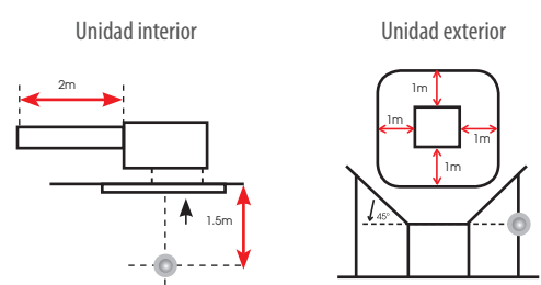
Medición presión sonora - Standard JIS B8616-2006
