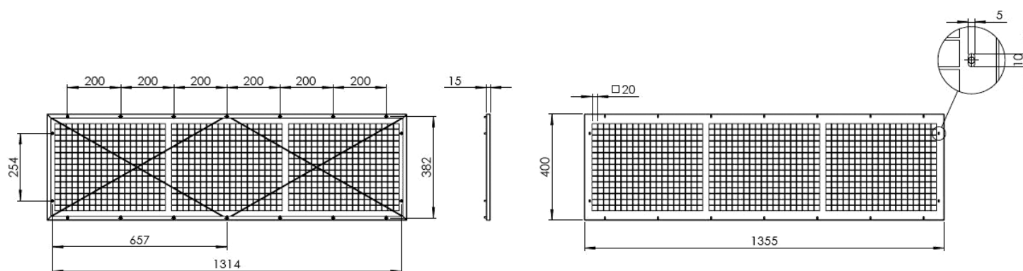
DETALLE B ESCALA 1 : 3
