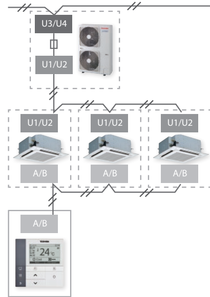
Grupo de unidades interiores
