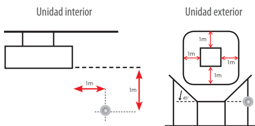
Medición presión sonora - Standard JIS B8616-2006
