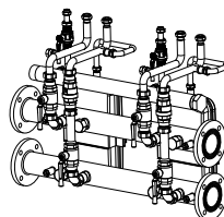
Kit hidráulico doble (para 2 calderas)
