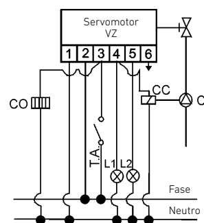
Conexiones eléctricas
